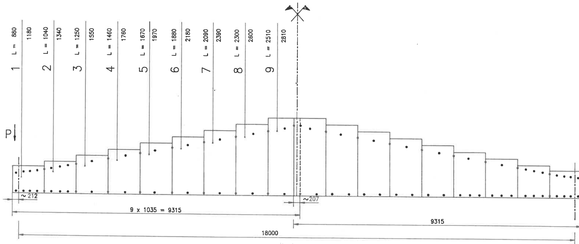
POHLED "P"
