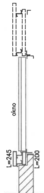
ŠTÍTOVÁ STĚNA
