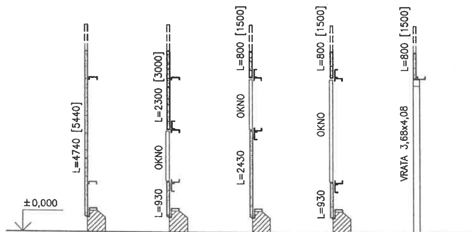
PODÉLNÁ STĚNA
