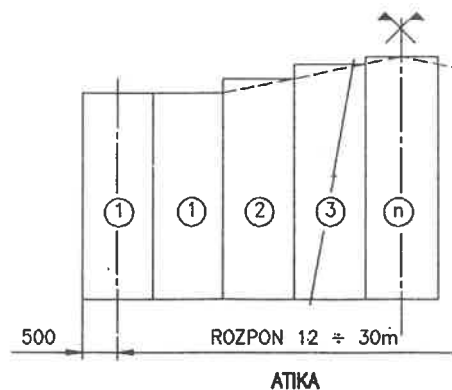
ATIKA
