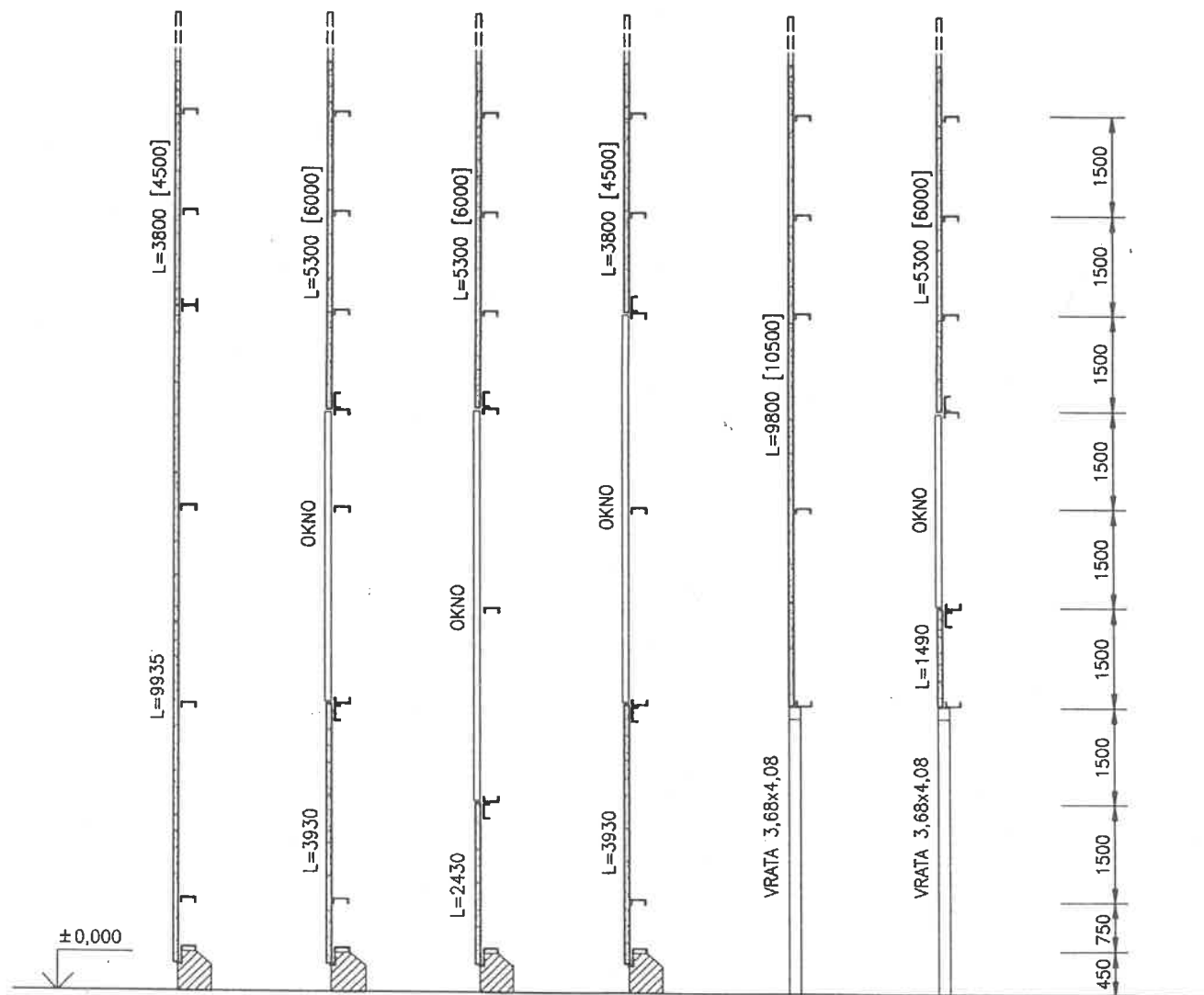
PODÉLNÁ STĚNA
