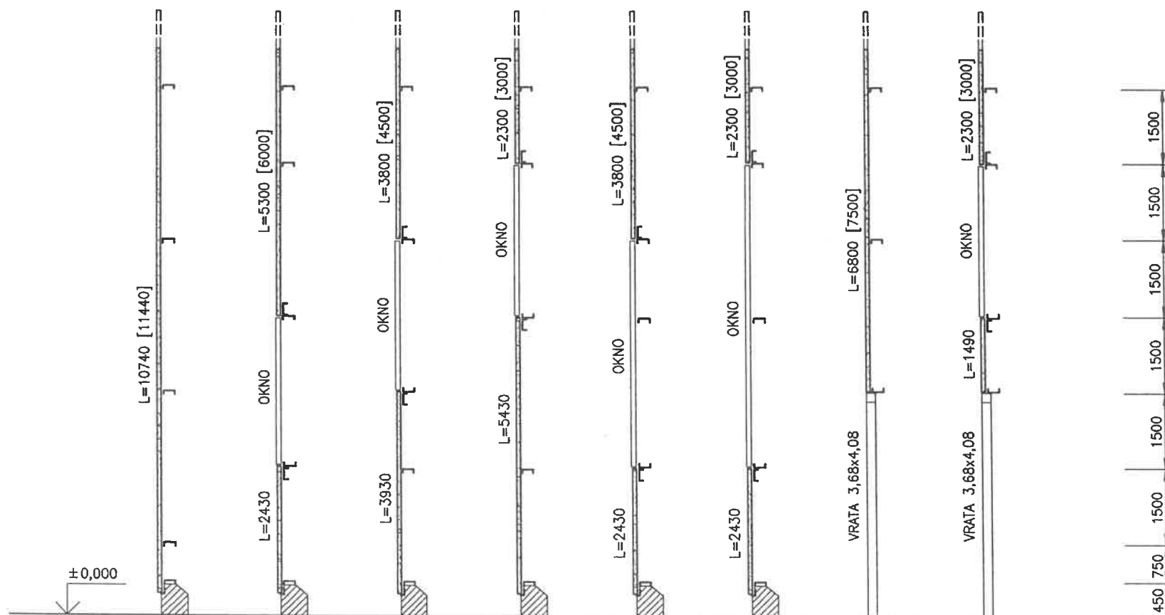
PODÉLNÁ STĚNA
