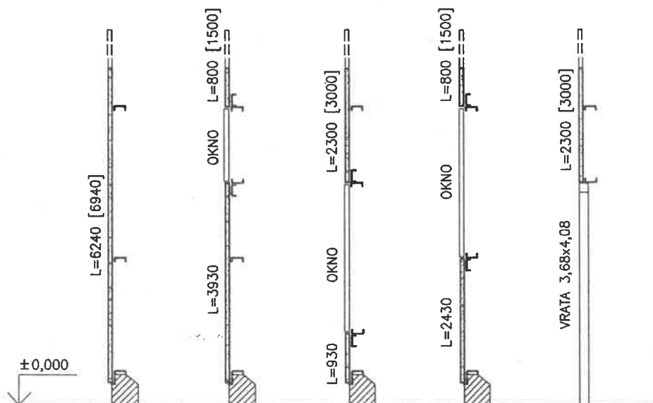
PODÉLNÁ STĚNA
