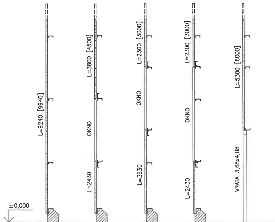
PODÉLNÁ STĚNA
