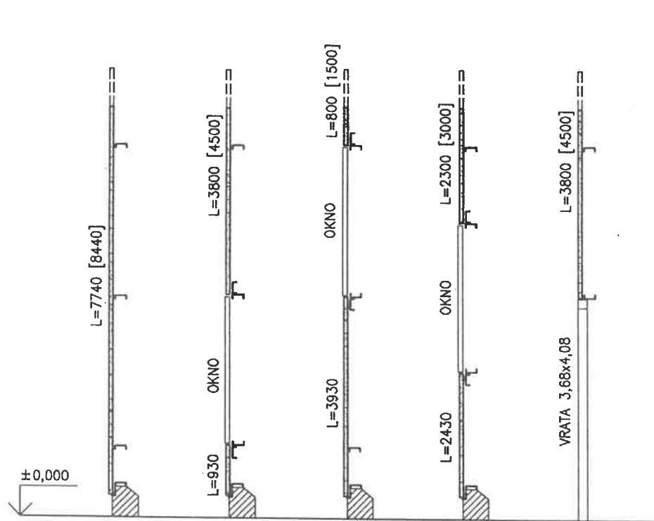
PODÉLNÁ STĚNA
