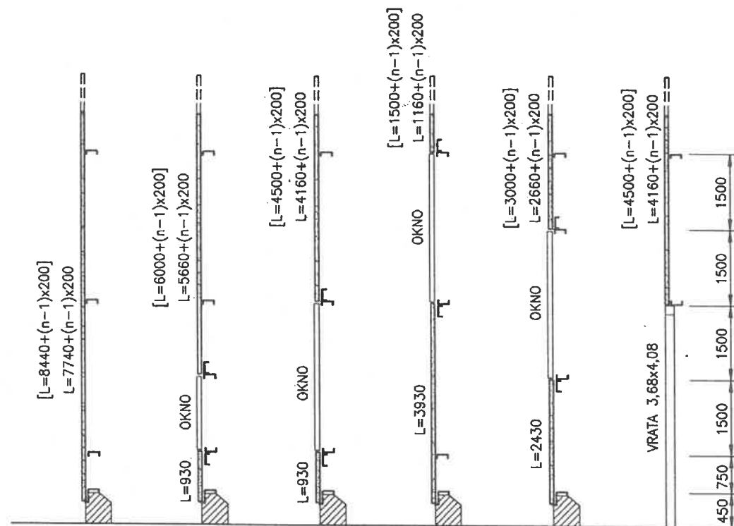
ŠTÍTOVÁ STĚNA
