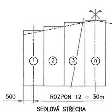
SEDLOVÁ STŘECHA
